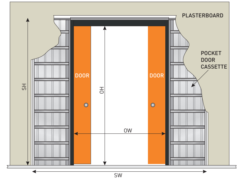
Double Pocket Door – Size Guide
